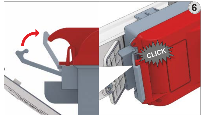
Deckel verriegeln.
