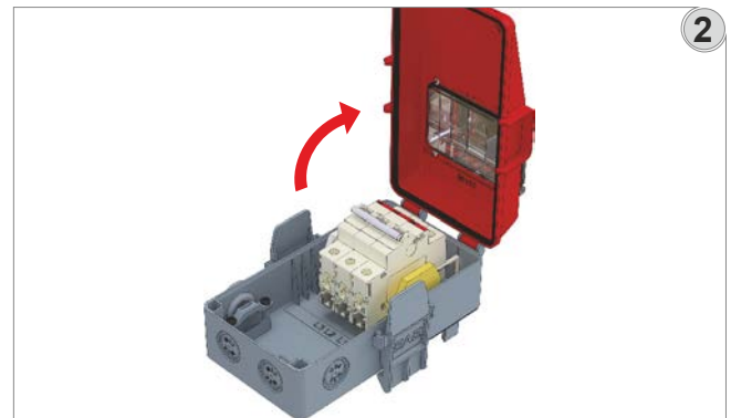
2- Deckel öffnen.
