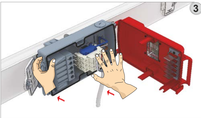
Kabelanschluss vornehmen.
