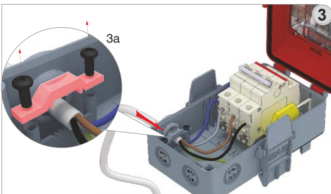
3- Kabelanschluß vornehmen.
